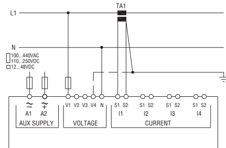
Connessione monofase con o senza V4 P01.07 = L1-N
