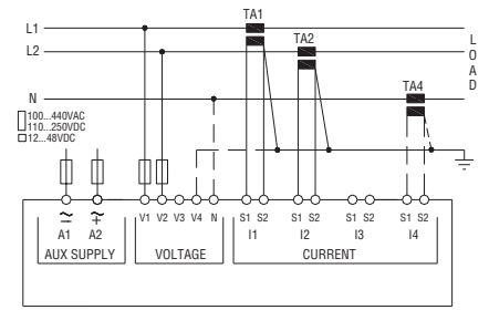
Connessione bifase con o senza V4 e corrente di neutro P01.07 = L1-N-L2
