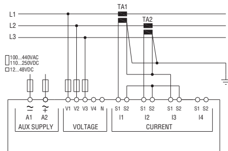
Connessione ARON 3 fasi senza neutro, con o senza V4 P01.07 = L1-L2-L3
